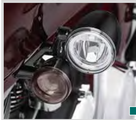
D. MONTAGEKIT FÜR ROAD GLIDE LED-NEBELSCHEINWERFER – SCHWARZGLÄNZEND
